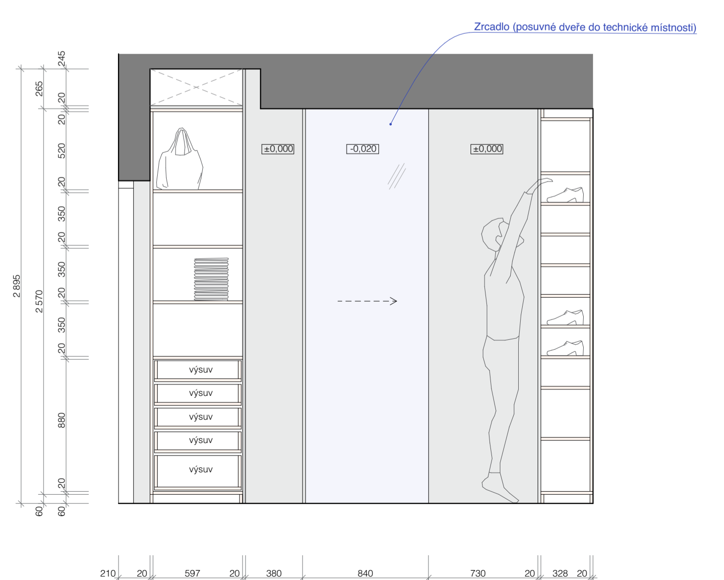
POHLED 2 - VNITŘNÍ ČLENĚNÍ SKŘÍNĚ
