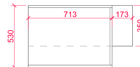
POHLED SHORA - s přebal. pultem
