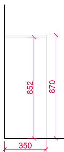
BOČNÍ POHLEDY s obdél. deskou
