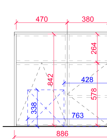
POHLED SHORA - s obdél. deskou
