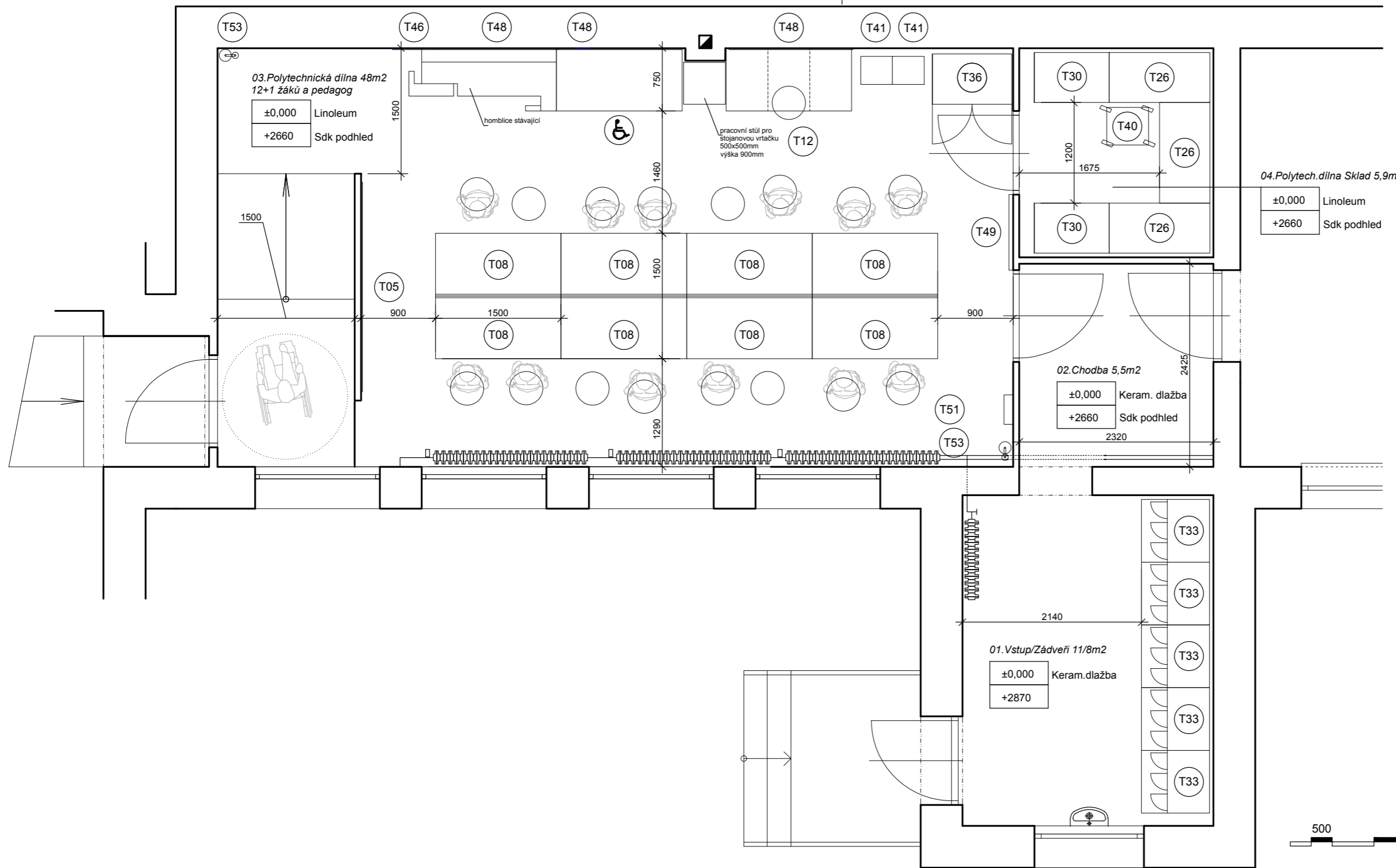
LEGENDA MÍSTNOSTÍ 1.NP
