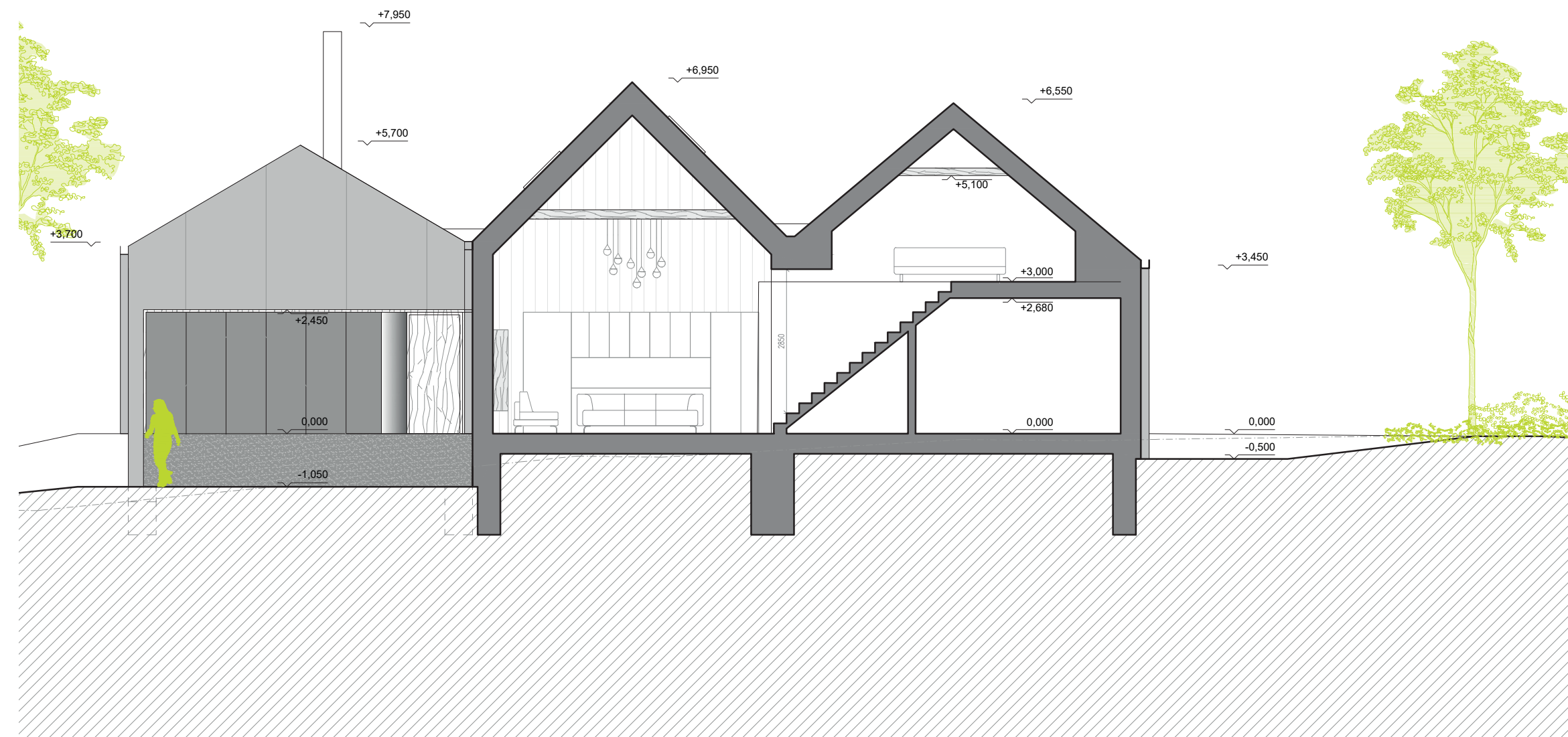
ŘEZ A-A
