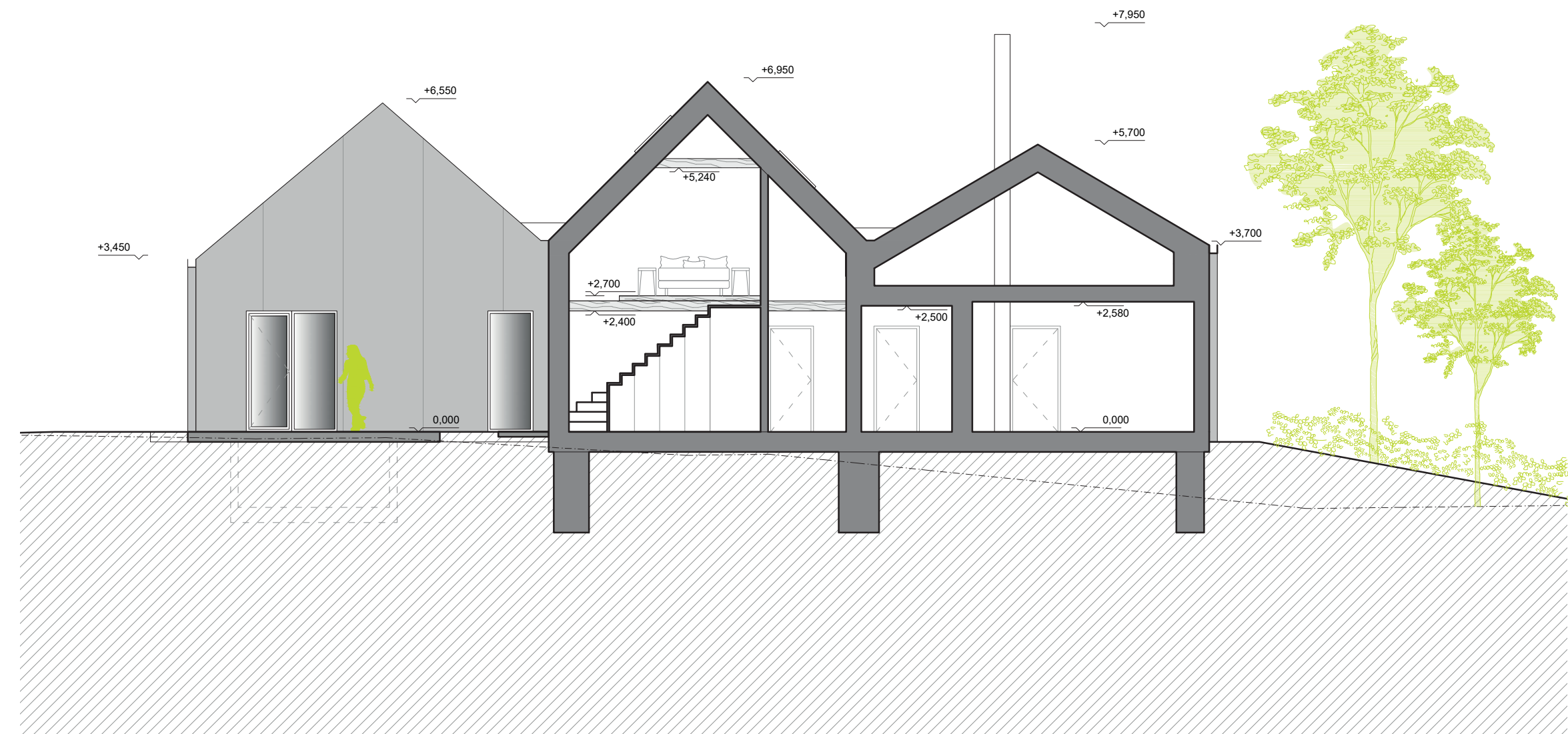
ŘEZ B-B
